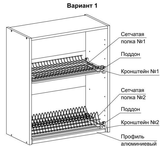
Схема 2. Варианты установки сетчатых полок
