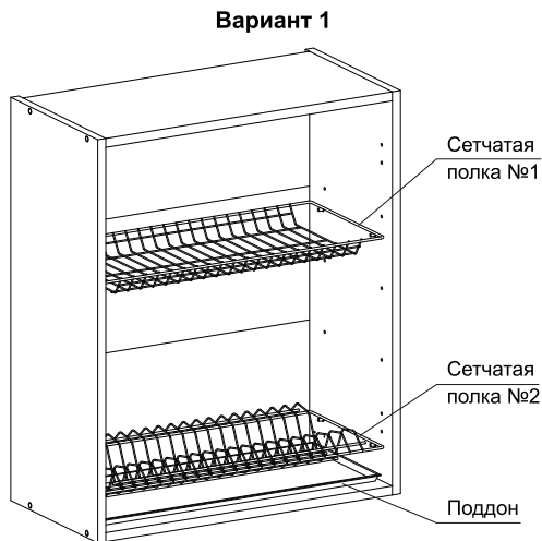
Схема 2. Варианты установки сетчатых полок
