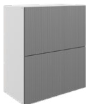
Шкаф навесной (2 двери горизонт.) → 1 711 ↑ 600|314|720
